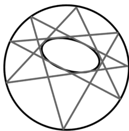
FIGURE 20.8. Poncelet’s Porism 20.10.8
